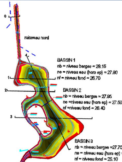
Modélisation 3D de la rivière et du lac – SODEREF – Janvier 2016
